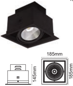
Cora 19 20W
