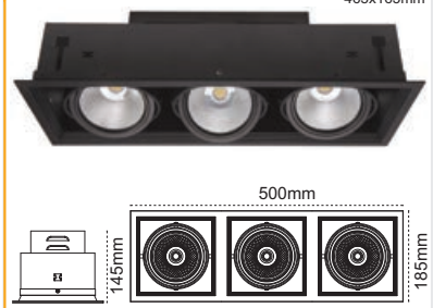
Cora 19 3X20W
