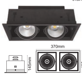
Cora 19 2X20W
