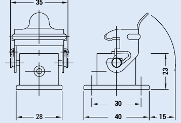
Montaj Eksenleri (22x22)
